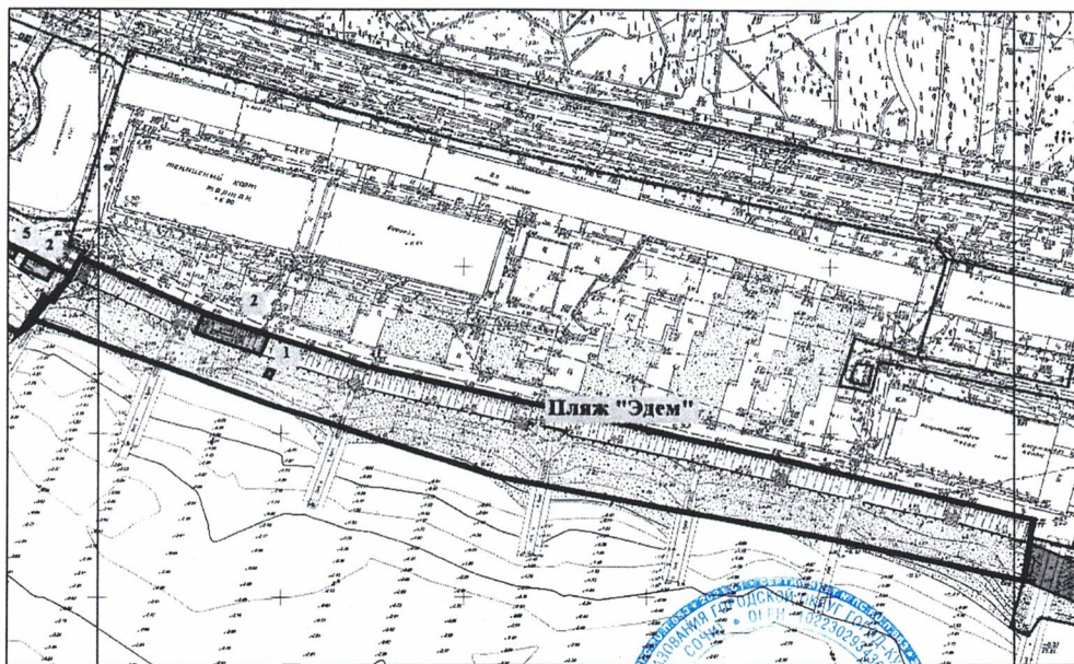
Пляж «Эдем» (L - 280 м, S – 5 742 м2), Хостинского внутригородского района муниципального образования городской округ город-курорт Сочи Краснодарского края (графическая часть, М 1:1000)
